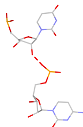
U:C pS(sp:O2*-O1P)
