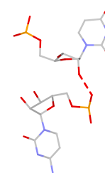
U:C rS(sp:O2*-O2P)
