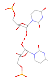
U:C rpS(ss:O2*-O2*)_1
