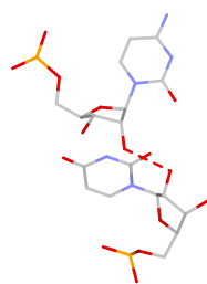
U:C fS*(ss:O2*-O2*)
