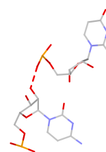
U:C rpS(ps:O2P-O2*)
