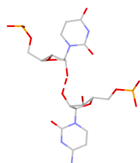
U:C rS(ss:O2*-O2*)
