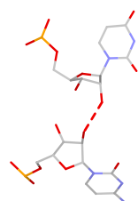
U:C rpS(ss:O2*-O2*)_2
