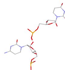
U:C rS(ps:O2P-O2*)
