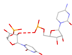
U:C pS*(sp:O2*-O1P)
