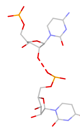
U:C pS*(ps:O1P-O2*)
