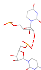
U:C pS(sp:O2*-O2P)
