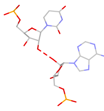
U:A rpS(ss:O2*-O2*)_1
