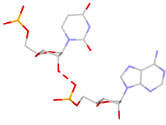
U:A pS(sp:O2*-O2P)
