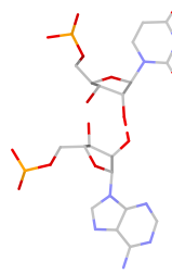
U:A rpS(ss:O2*-O2*)_2
