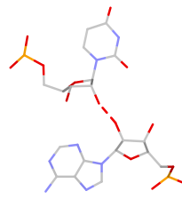
U:A rS(ss:O2*-O2*)_1
