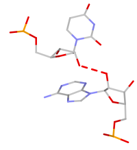
U:A rS(ss:O2*-O2*)_2
