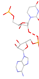
U:A rS(sp:O2*-O1P)
