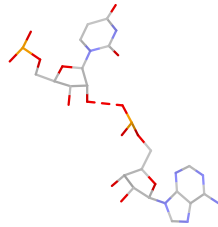
U:A rpS(sp:O2*-O1P)
