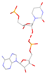
U:A S(sp:O2*-O2P)
