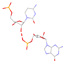
C:G rpS(sp:O2*-O1P)
