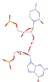
C:G rpS(ss:O2*-O2*)
