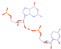
C:G pS*(ps:O1P-O2*)
