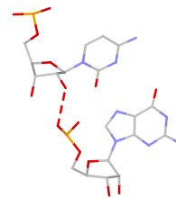
C:G pS(sp:O2*-O2P)
