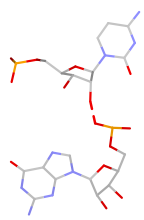
C:G S(sp:O2*-O2P)
