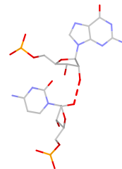
C:G fS*(ss:O2*-O2*)
