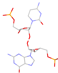
C:G rS(ss:O2*-O2*)
