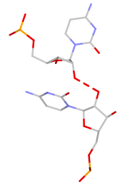
C:C rS(ss:O2*-O2*)_2
