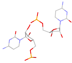
C:C rS(ps:O1P-O2*)
