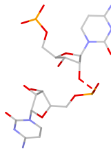
C:C rS(sp:O2*-O2P)
