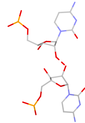
C:C rpS(ss:O2*-O2*)
