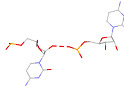
C:C rpS(ps:O2P-O2*)
