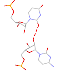
U:C rpS(bs:O2-O2*)
