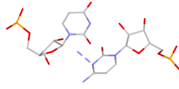
U:C rS(bs:N3-O2*)
