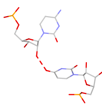
U:C S*(pb:O2P-N4)
