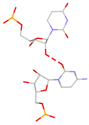
U:C rpS(sb:O2*-O2)
