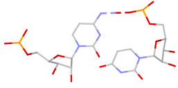
U:C S*(pb:O2P-N4)
