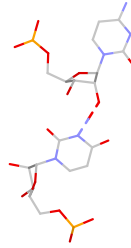
U:C pfS*(bs:N3-O2*)
