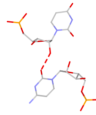
U:C rS(sb:O2*-O2)
